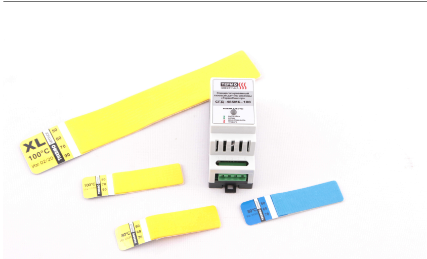
Рисунок 69 Газовыделяющие наклейки системы "термосенсор" с датчиком газа. Корпус датчика – обычный DIN-модуль на рейку.
